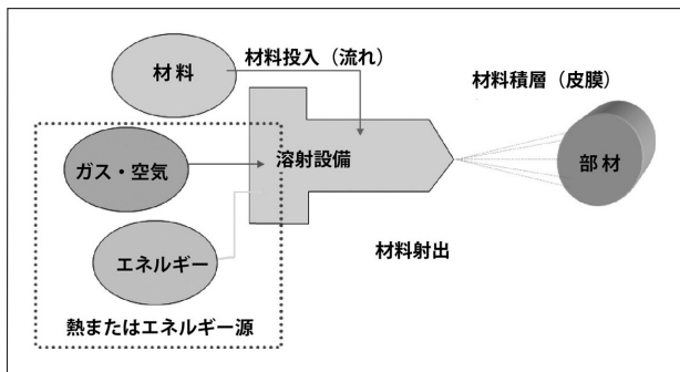
図2a 溶射における熱・エネルギー源の要件
