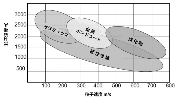
図4b 異なる材料系における粒子温度と粒子速度の関係
