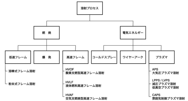
図3 溶射プロセスの種類 (HVOF: 酸素支燃型高速フレイム溶射, HVLFF: 液体燃料高速フレイム溶射, HVAFF: 空気支燃型高速フレイム溶射, APS: 大気圧プラズマ溶射, LPPS/LVPS: 減圧プラズマ溶射 / 低真空プラズマ溶射, CAPS: Controlled Atmospheric Plasma Spray (雰囲気制御プラズマ溶射))
