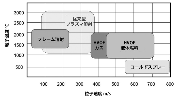
図4a 溶射プロセスにおける粒子温度と粒子速度の関係
